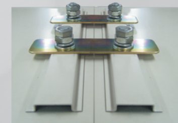
● キャビネット連結工事例
