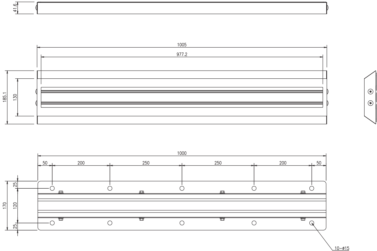
垂直面用アルミレール縦横兼用設置L1000mmタイプ (型番:FTK-XYA1000)
