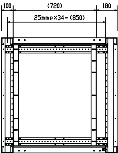
側面断面図
