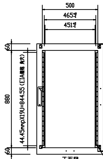
正面図 (扉を外した状態) マウントアングル (EIA規格 ケージナット仕様) (U表示付)
