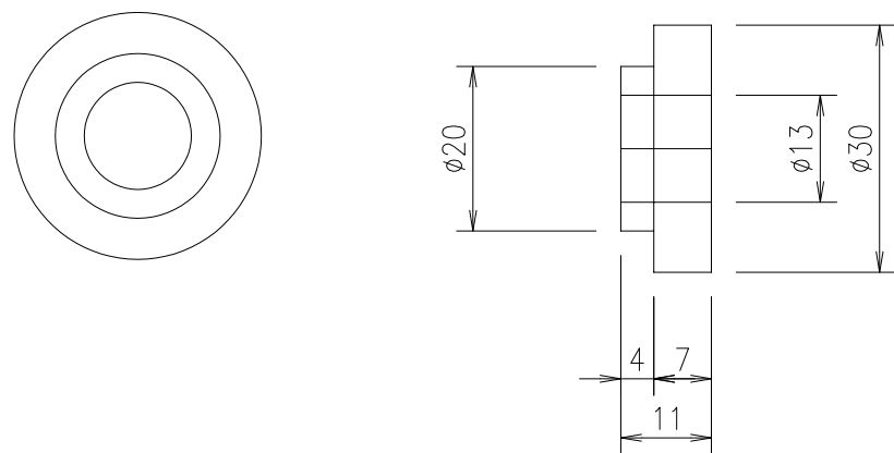
絶縁ブッシング (4B-KD20)
