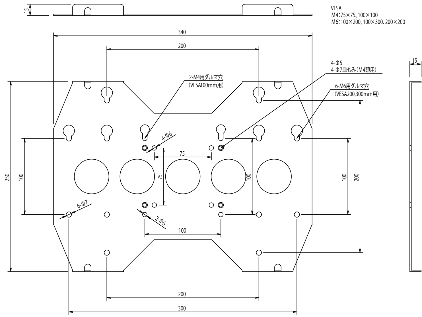
クレーンアームVESA変換金具 (型番:FFP-TP)
