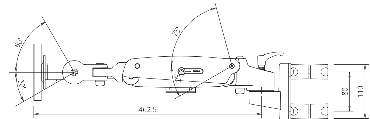
クレーンアーム本体-ポールクランプ付垂直ベース-簡易ロック有り(型番:FFP-QAL-PBL)
