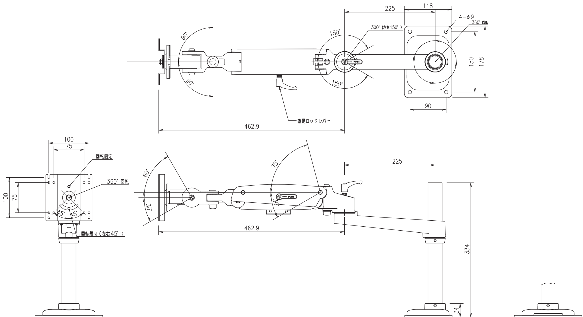
クレーン-ム-本体-直付デスクベース-延長アーム-簡易ロック有り(型番:FFP-QAL-DDB-EFL)
