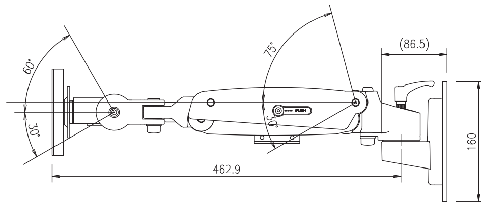
クレーンアーム本体-直付垂直ベース-簡易ロック有り(型番:FFP-QAL-DBL)
