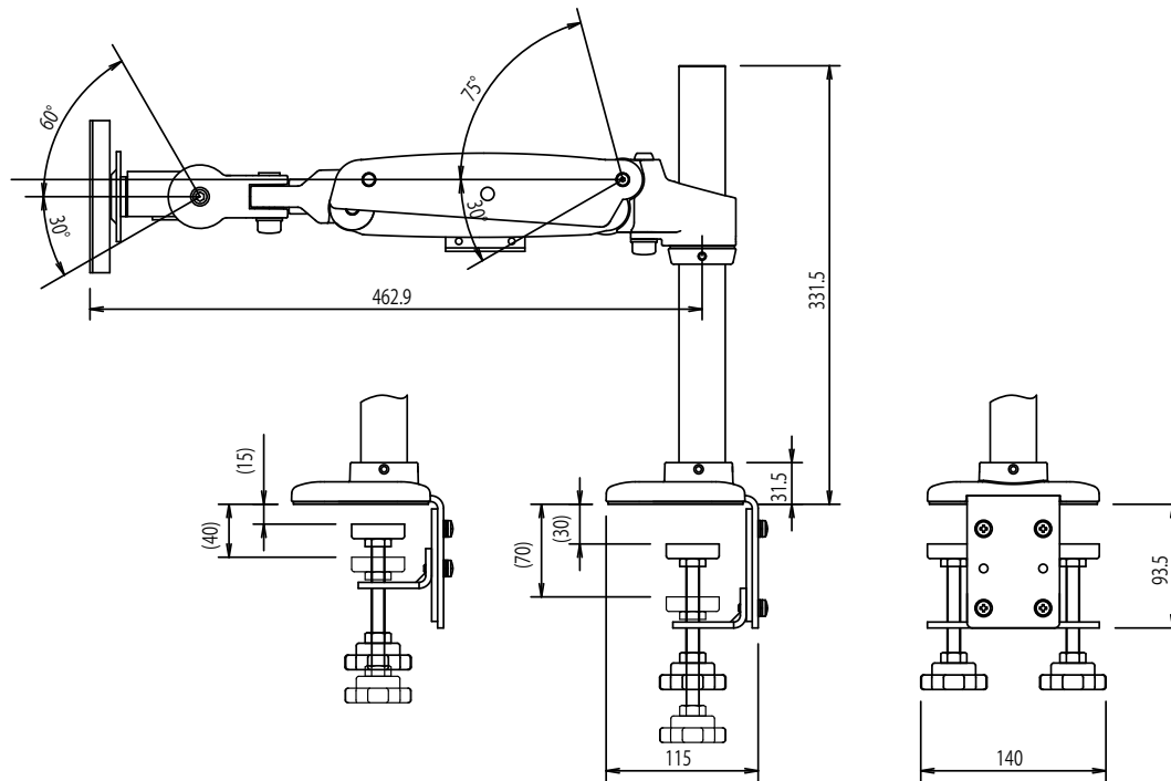
クレーン-ム-本体-デスククランプ-簡易ロック無し (型番:FFP-QA-DC)
