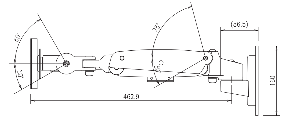
クレーンアーム本体-直付垂直ベ-ス-簡易ロック無し(型番:FFP-QA-DB)
