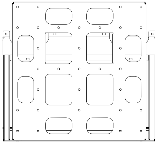
正面図
