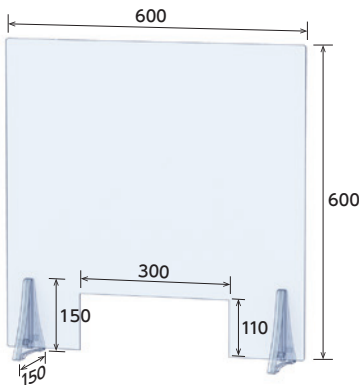
【型番: FFP-HAS-66】
