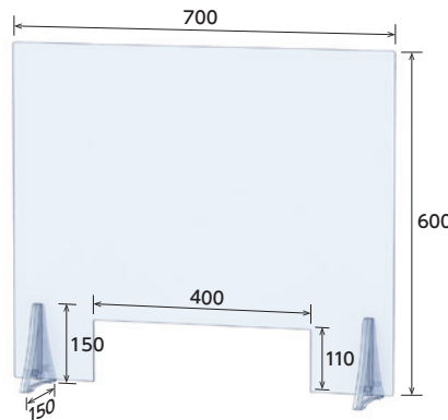
【型番: FFP-HAS-76】
