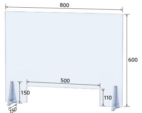
【型番: FFP-HAS-86】
