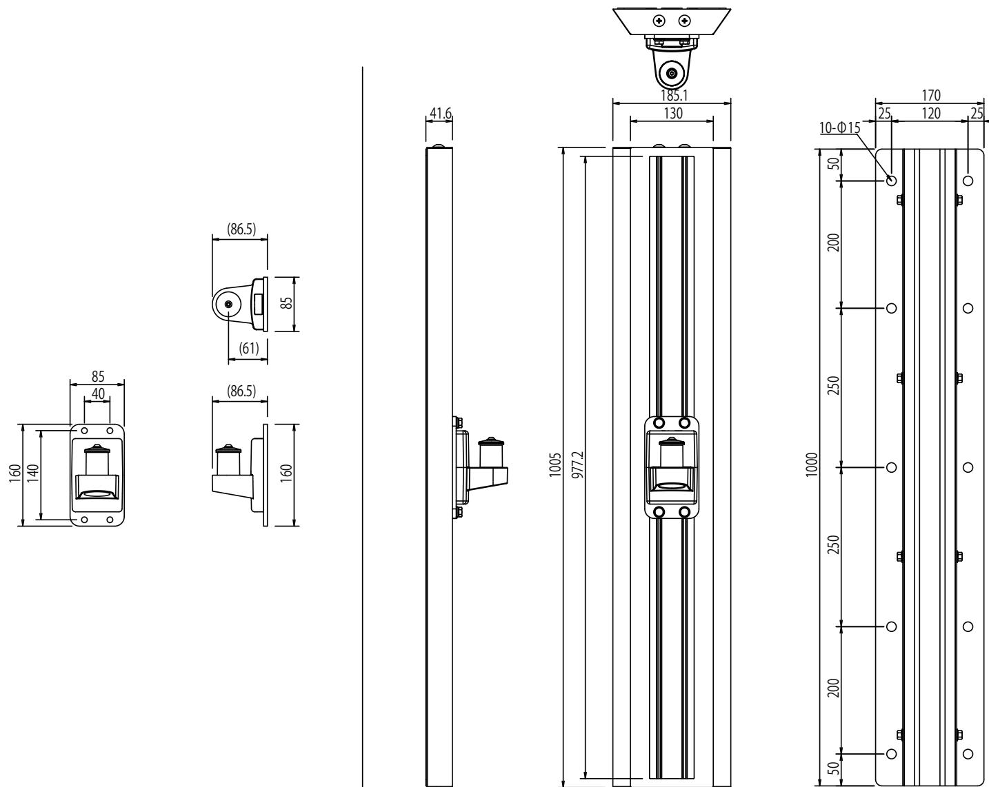
クレーンアーム縦型壁面用アルミレールレバー無し(型番:FFP-AH1000)
