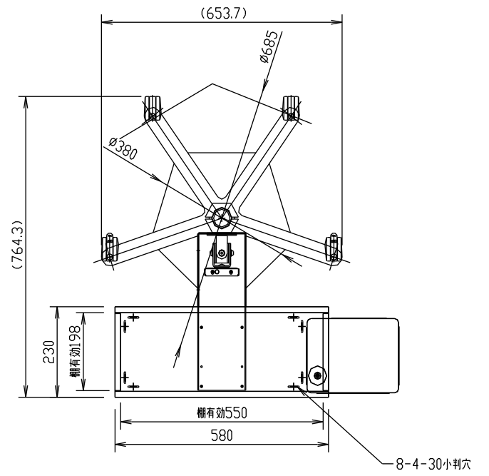
A-A 矢視図
